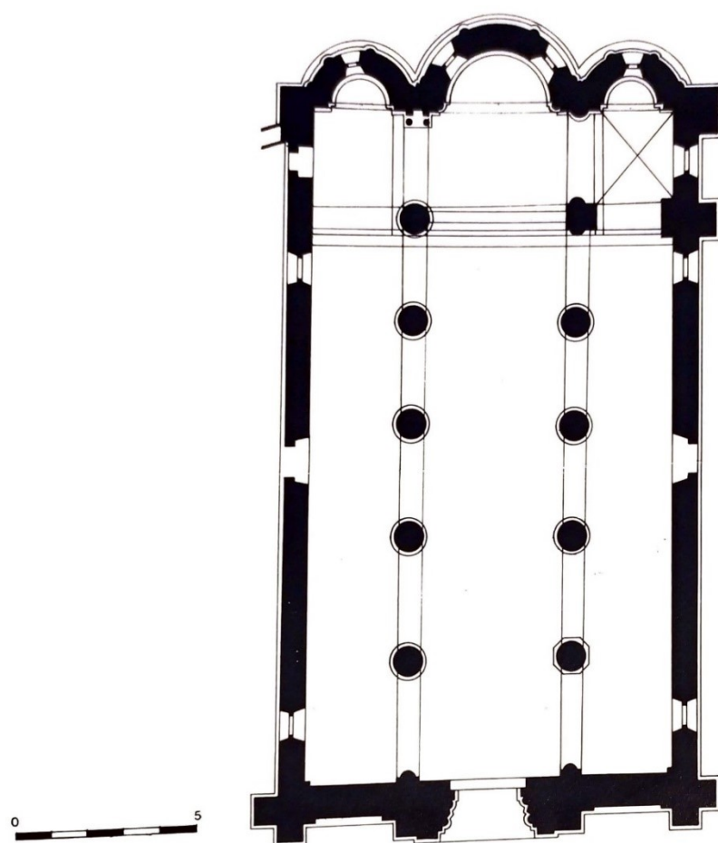
Fig. 359 – Vigoleno (PC), pieve di San Giorgio – planimetria (da SEGAGNI 1984a, p. 541)
