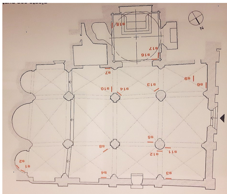
Fig. 118 – Piacenza, chiesa di Santa Brigida – planimetria stato attuale Su gentile concessione della SABAP-Pr (cart. PC/M 12 – rilievo 2013)
