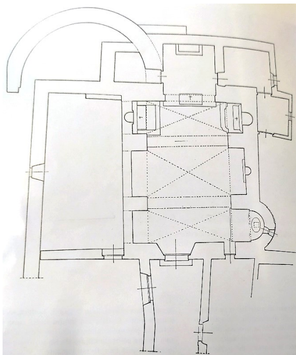
Fig. 302 – Monteventano (Piozzano, PC), chiesa di Santa Maria presso il Castello – rilievo planimetrico (arch. L. Summer, tratto da SUMMER 1990, p. 58, fig. 31)
