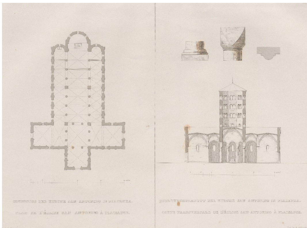
Fig. 136 – Piacenza, chiesa di Sant’Antonino – planimetria e rilievi (da OSTEN 1846)
