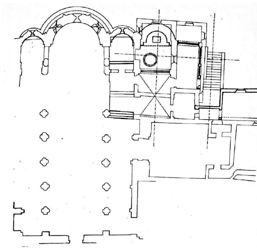
Fig. 314 – Castell'Arquato (PC), collegiata di Santa Maria – planimetria della chiesa e degli annessi sud durante i restauri, 1912 (con indicazione della collocazione dei resti del battistero e della loggetta) (da VENEZIANI 1991, p. 249)
