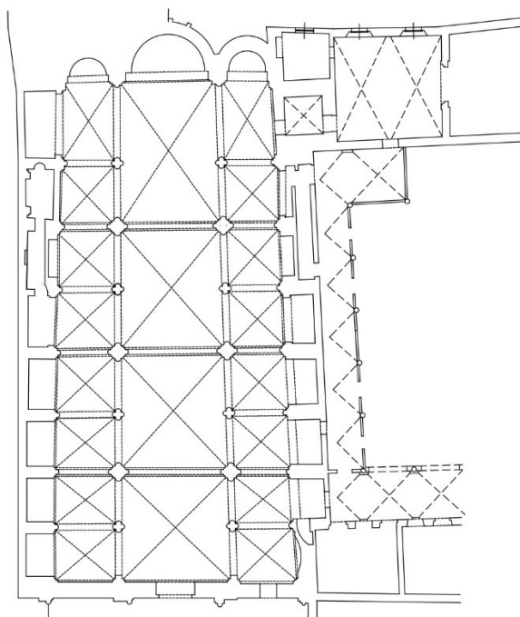
Fig. 34 – Piacenza, chiesa di Sant'Eufemia – planimetria (rilievi e disegno del geom. Ernesto Ferrari)
