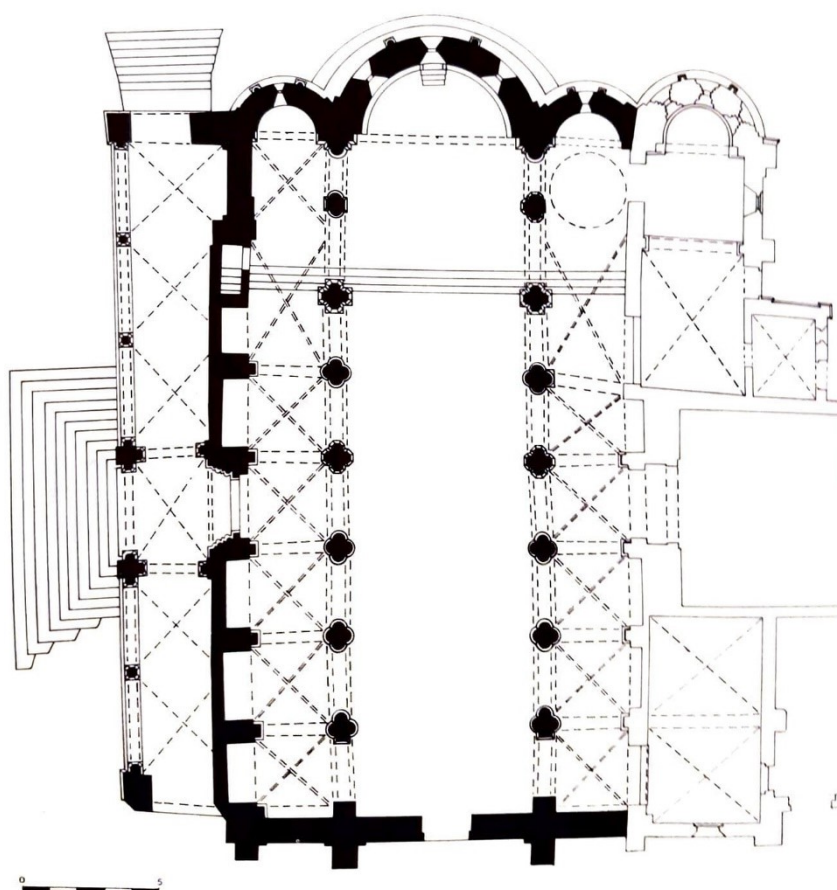
Fig. 313 – Castell'Arquato (PC), collegiata di Santa Maria – planimetria (da SEGAGNI 1984a, p. 498)
