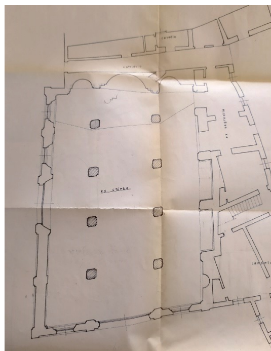
Fig. 193– Piacenza, demolita chiesa di Sant'Andrea in Borgo – planimetria 1957 Su gentile concessione della SABAP-Pr (cart. PC/M 98 – geom. Bolzoni)
