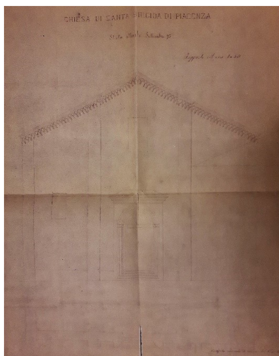
Fig. 120 – Piacenza, chiesa di Santa Brigida – rilievo dello stato della facciata prima del rifacimento, inizio XX secolo Su gentile concessione della SABAP-Pr (cart. PC/M 12)
