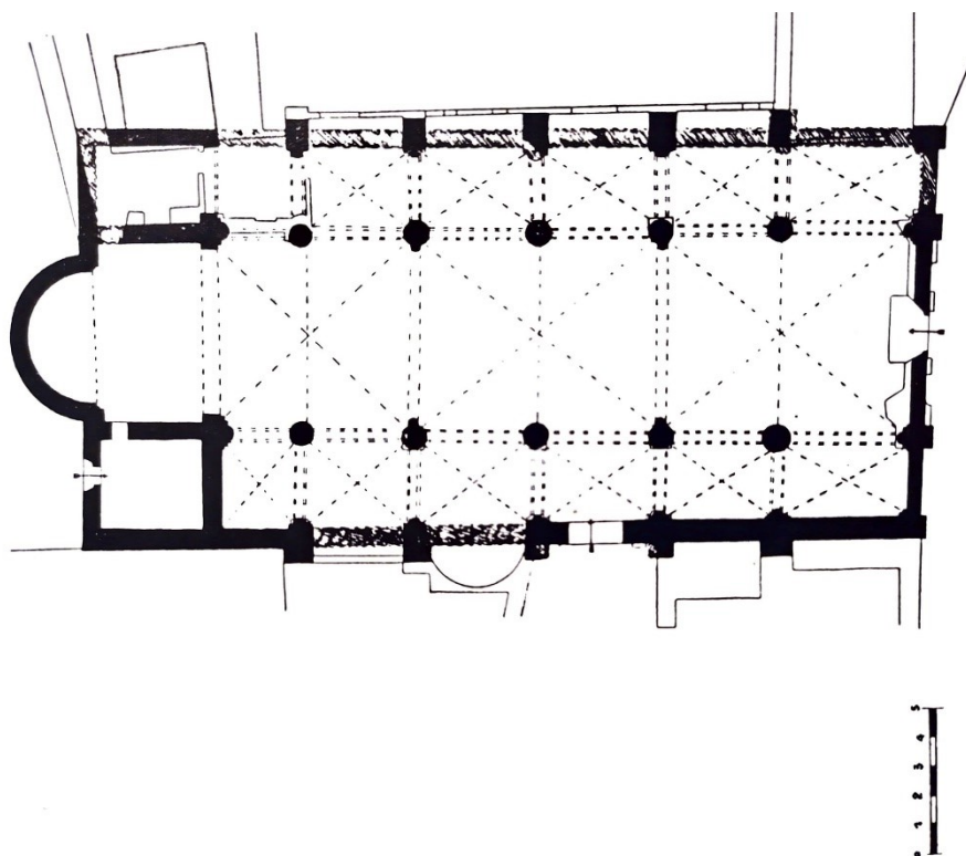
Fig. 166A – Piacenza, ex chiesa di San Matteo – planimetria (da ROMANINI 1951, p. 86)
