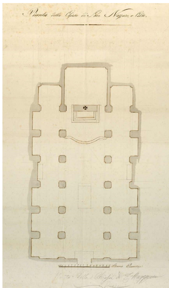
Fig. 201b – Piacenza, chiesa dei Santi Nazario e Celso – planimetria inizio XX secolo Su concessione del Ministero per i Beni e le Attività Culturali (ASPC, Fondo Mappe, stampe e disegni, n. 3916)
