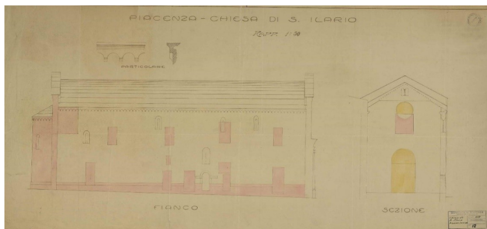
Fig. 218 – Piacenza, chiesa di Sant'Ilario – rilievi con indicazioni parti di restauro, 1928 Su concessione del Ministero per i Beni e le Attività Culturali (ASPC, Fondo Mappe, stampe e disegni, n. 5642)
