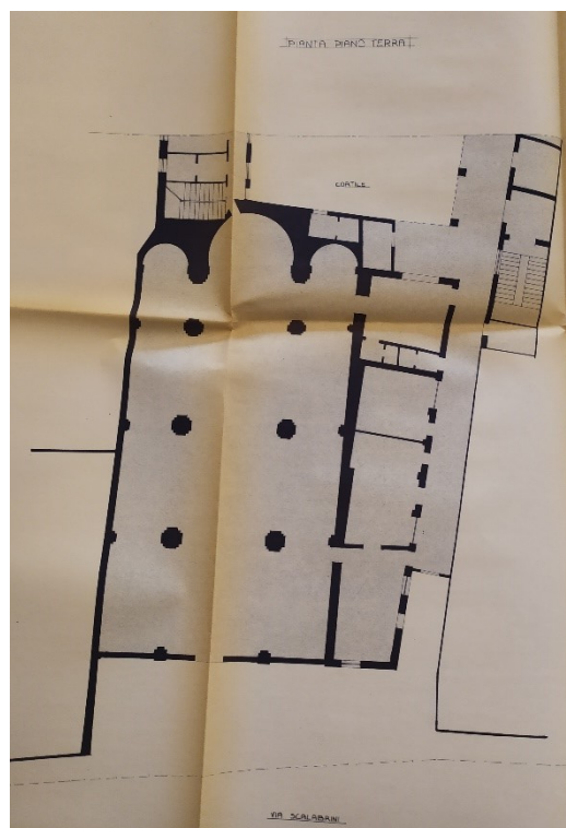
Fig. 155 – Piacenza, chiesa di Santo Stefano – planimetria, 1985 Su gentile concessione della SABAP-Pr (cart. PC/M 217, rilievo arch. C. Ferrari)
