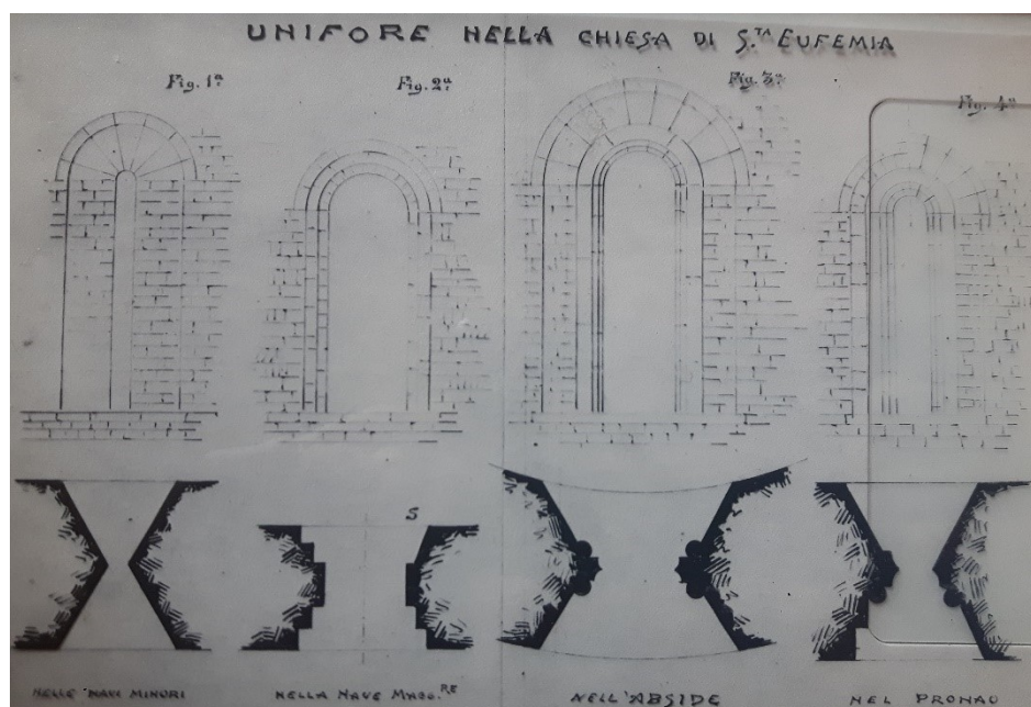
Fig. 31 – arch. Camillo Guidotti, rilievo su velina con profilo delle monofore della chiesa di Sant'Eufemia, marzo 1904 Su gentile concessione della SABAP-Pr (cart. PC/M 31)
