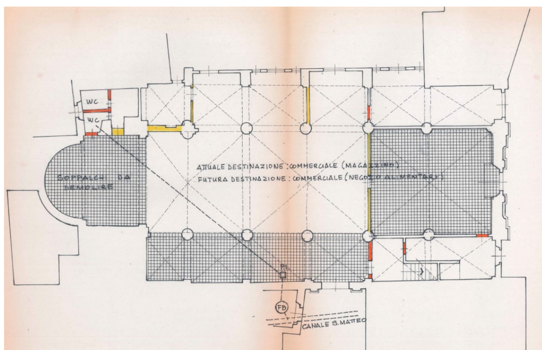
Fig. 166B – Piacenza, ex chiesa di San Matteo – planimetria anni '80 Su gentile concessione della SABAP-Pr (cart. PC/M 54)
