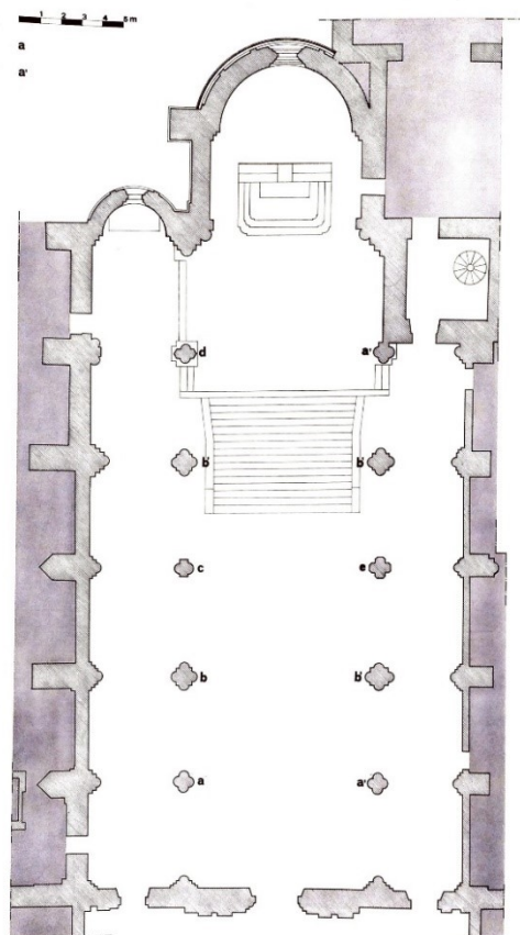
Fig. 65 – Piacenza, chiesa di San Savino – planimetria – chiesa superiore (da SALVINI 1978, p. 94)
