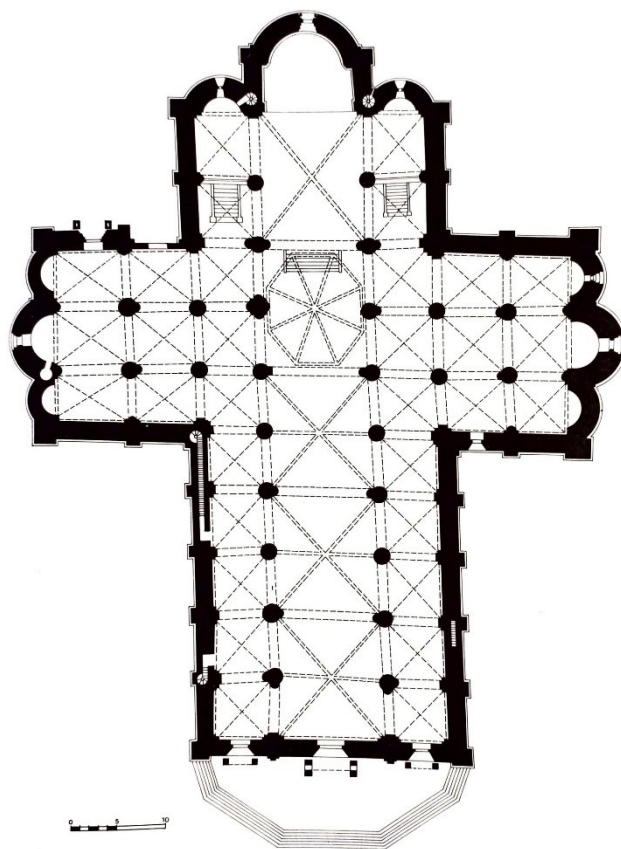
Fig. 11 - Piacenza, cattedrale di Santa Maria Assunta, planimetria (da SEGAGNI 1984a, p. 507)
