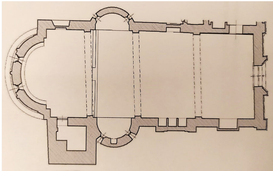
Fig. 279 - Breno (Borgonovo Val Tidone, PC), chiesa di Sant'Ilario – rilievo dello stato attuale dell'edificio (su gentile concessione dell'Archivio SABAP-Pr, cart. PC/M 178, tratto da "Progetto di restauro" arch. A. Bellocci, giugno 2010)
