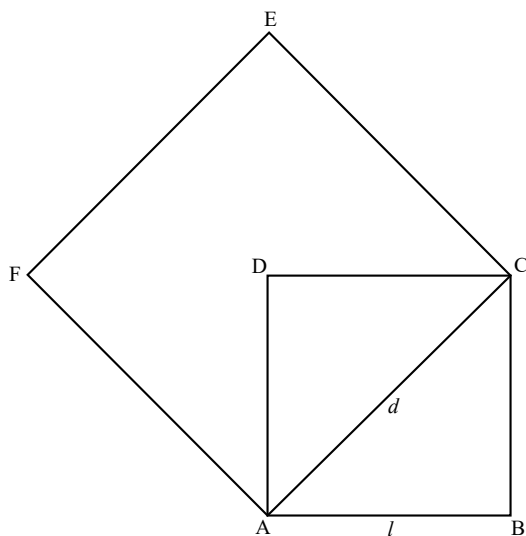
FIGURA 1 (In)commensurabilità di lato e diagonale nel quadrato
